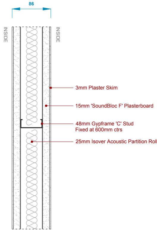
08 Type D Plan
