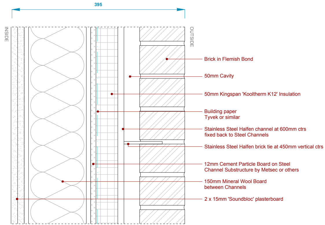
01 Type D : Brick / Steel Section
