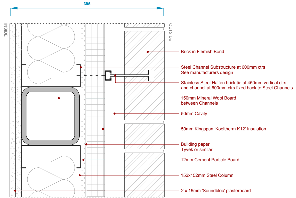
02 Type D : Brick / Steel Plan
