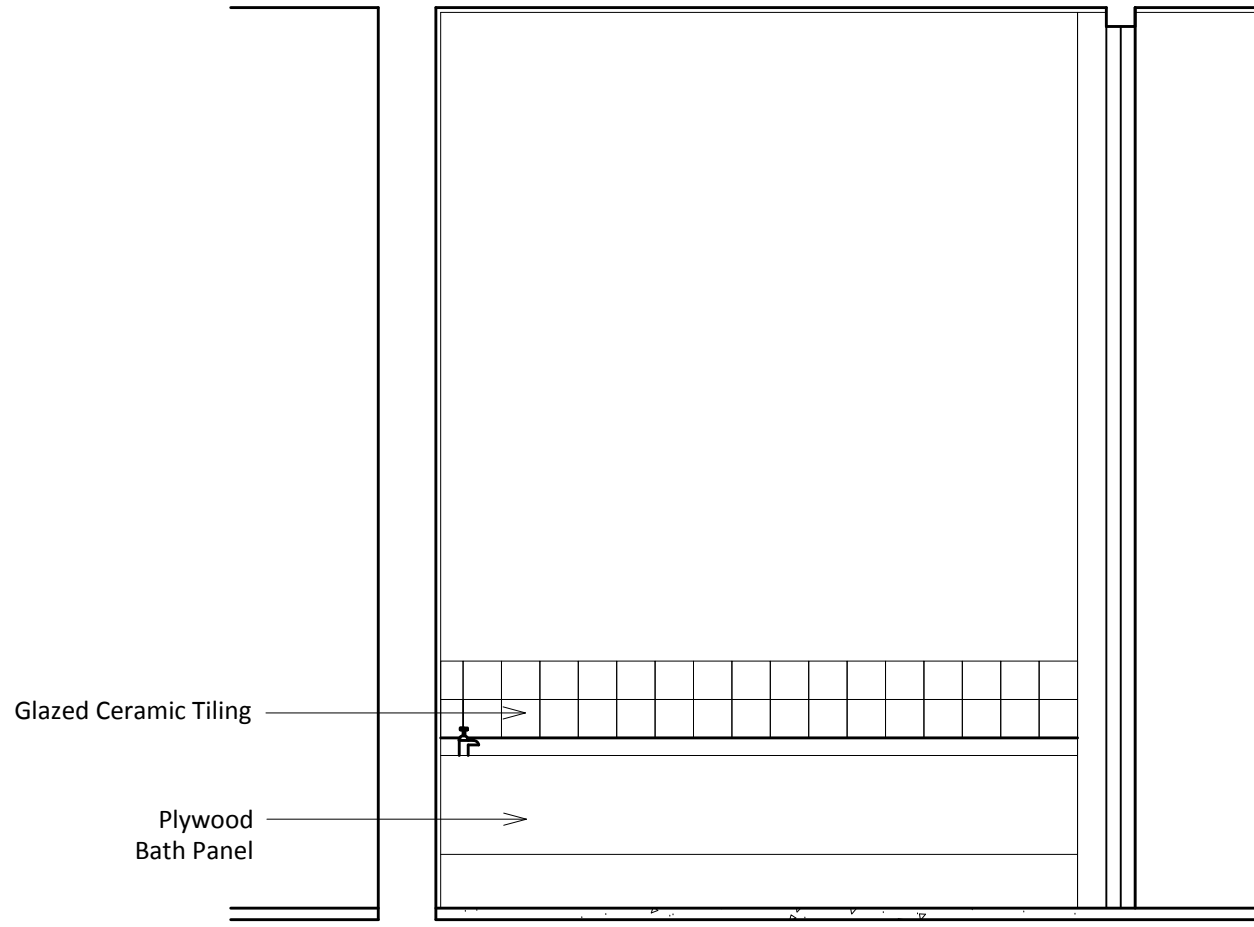
03 Section 02 207 1:20
