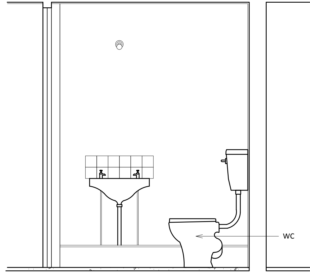
05 Section 04 207 1:20
