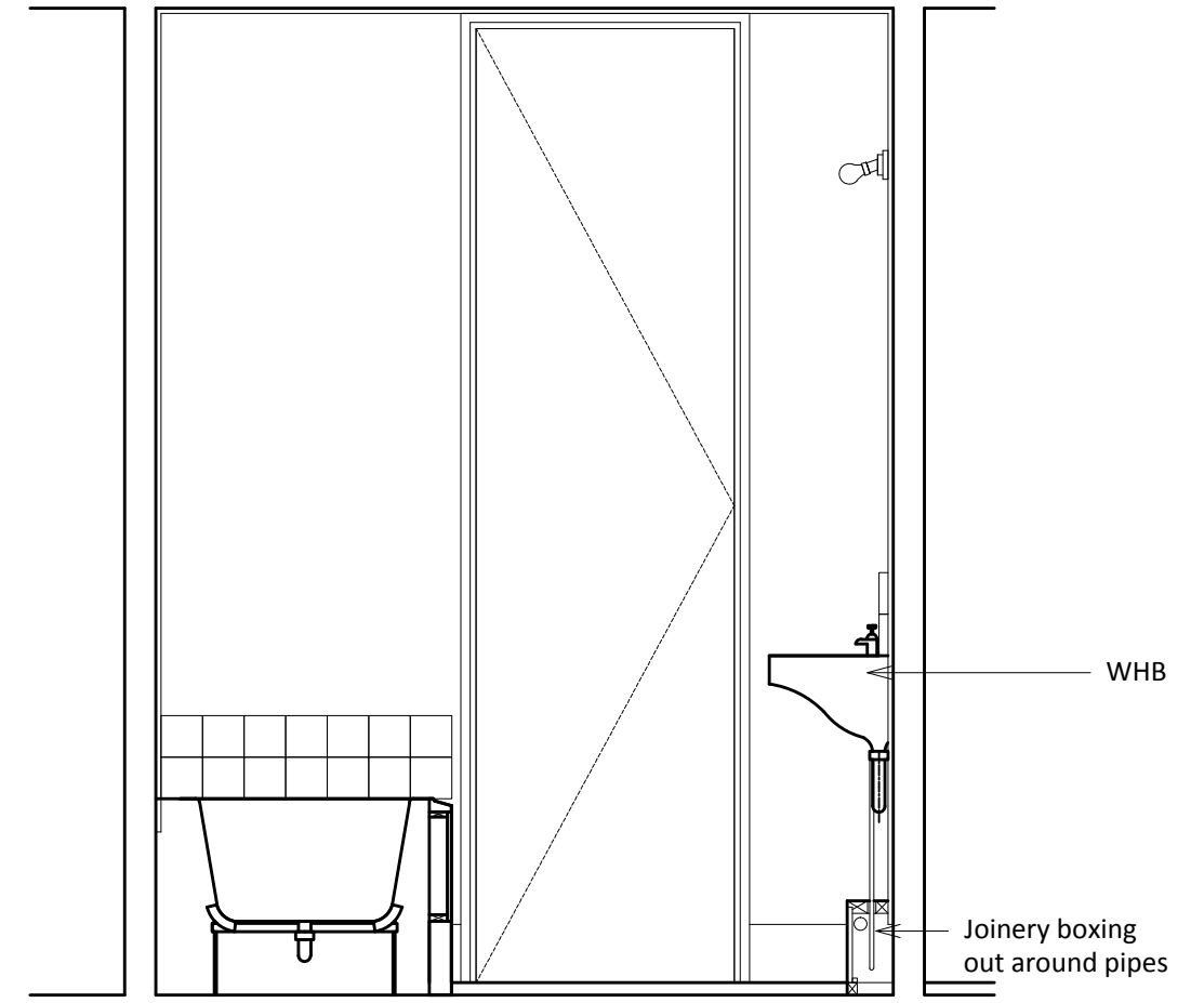
06 Section 05 207 1:20
