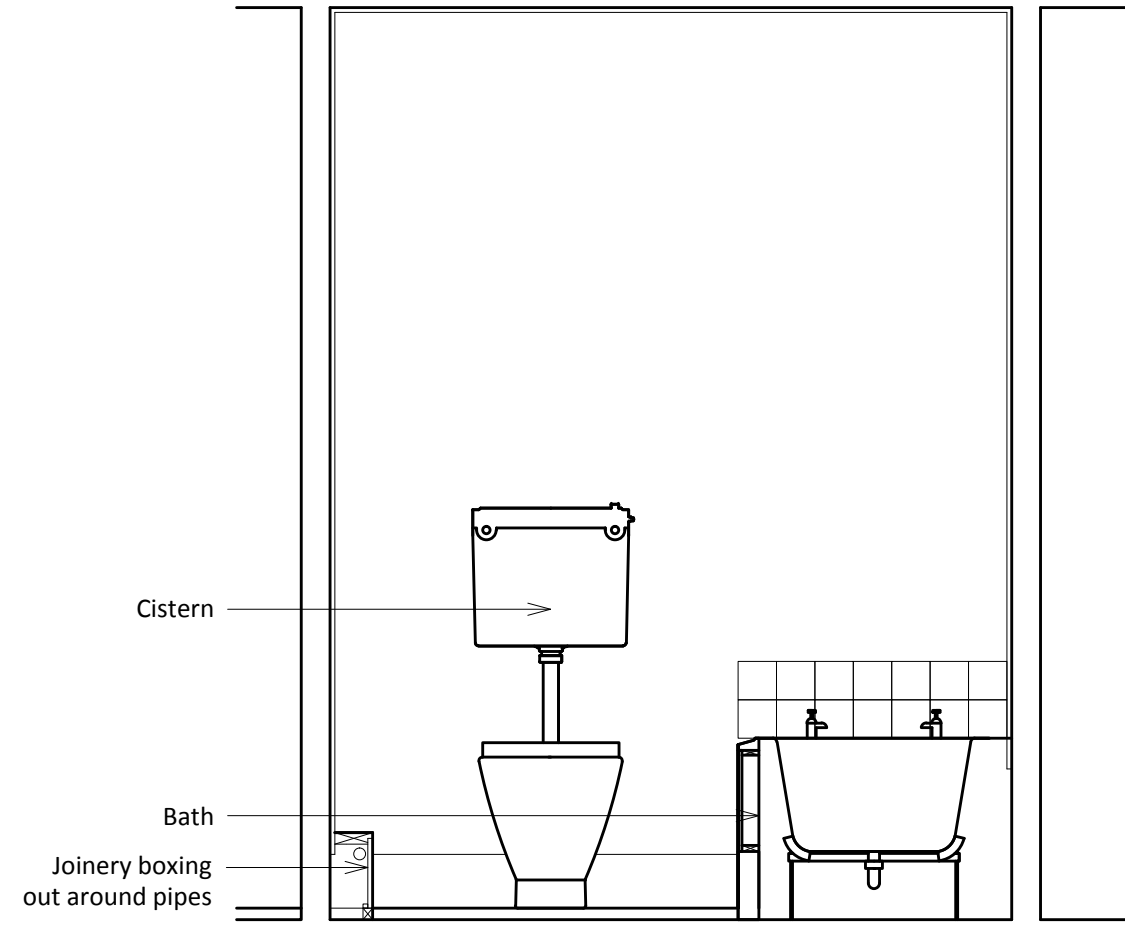
04 Section 03 207 1:20
