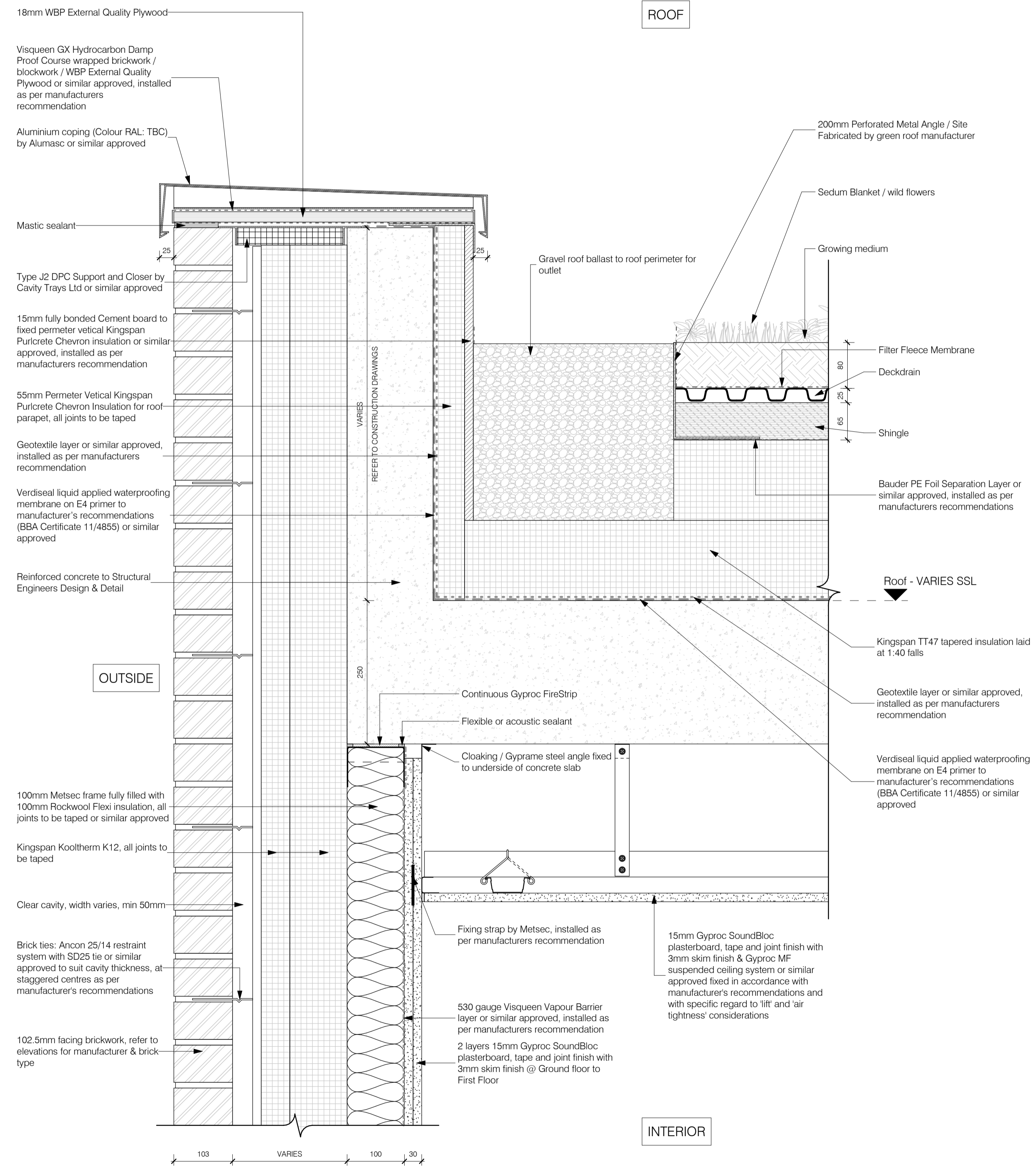
1 RWOS / SBM Scale: 1:5
