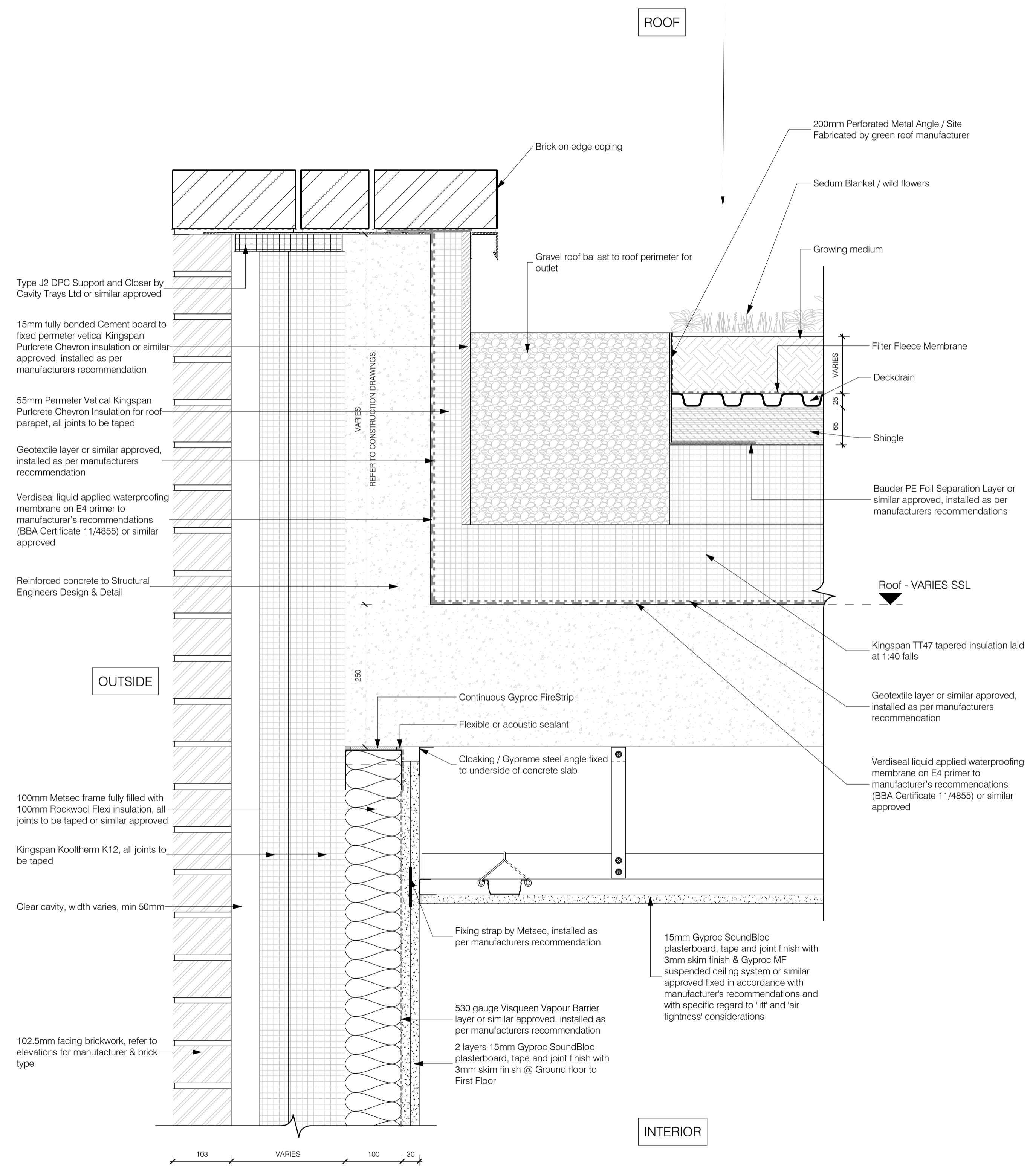
1 VARS lower roof Scale: 1:5
