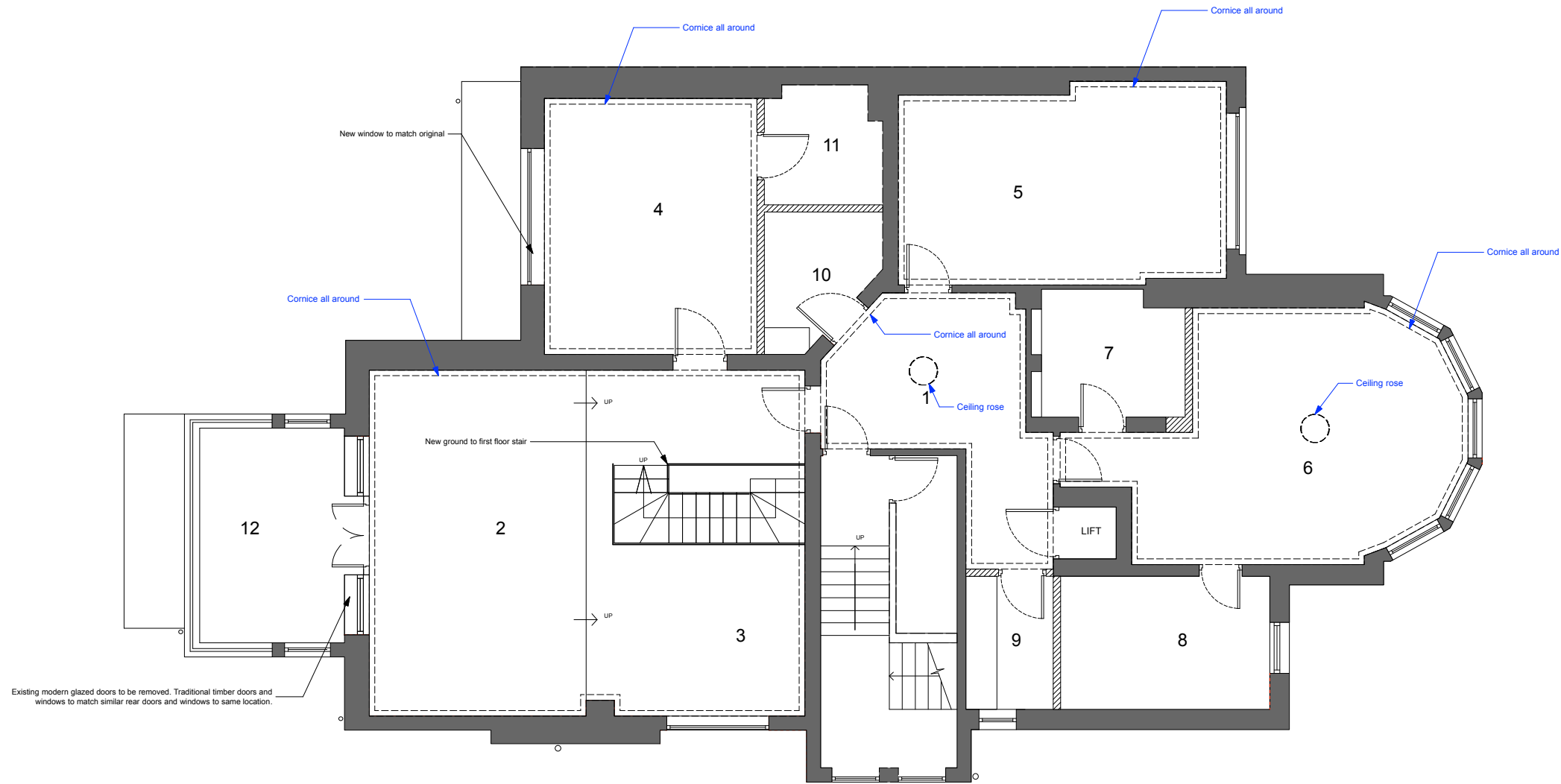
1 PLAN Scale: 1:50
