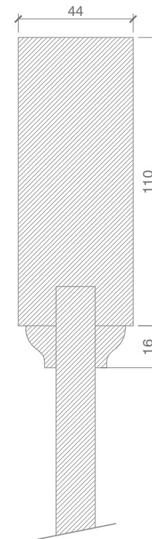
TYP. DOOR PROFILE DETAIL HIERARCHY 3 REGENCY FOUR PANEL DOOR SCALE - 1:2
