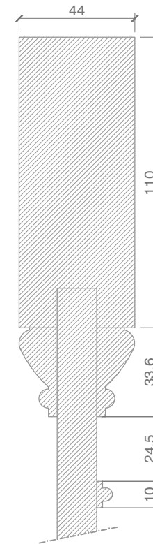
TYP. DOOR PROFILE DETAIL HIERARCHY 1 REGENCY FOUR PANEL DOOR SCALE - 1:2
