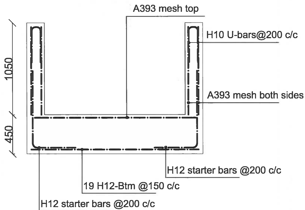
Section A-A 1:25
