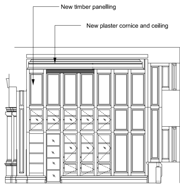
Elevation A
