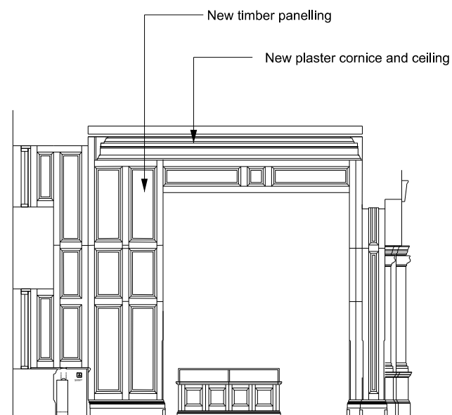
Elevation A
