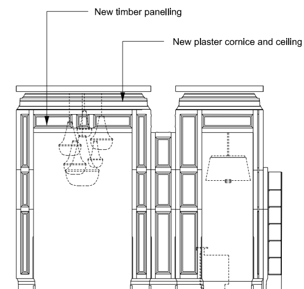
Elevation E
