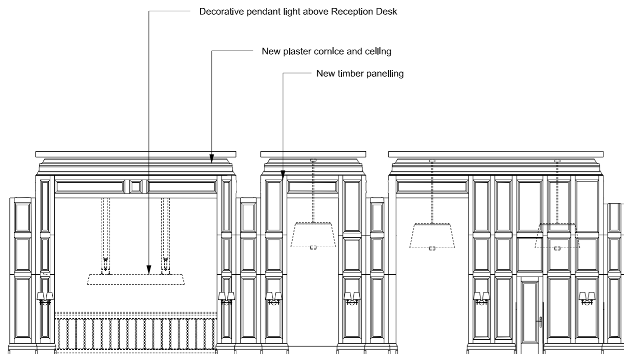
Elevation A
