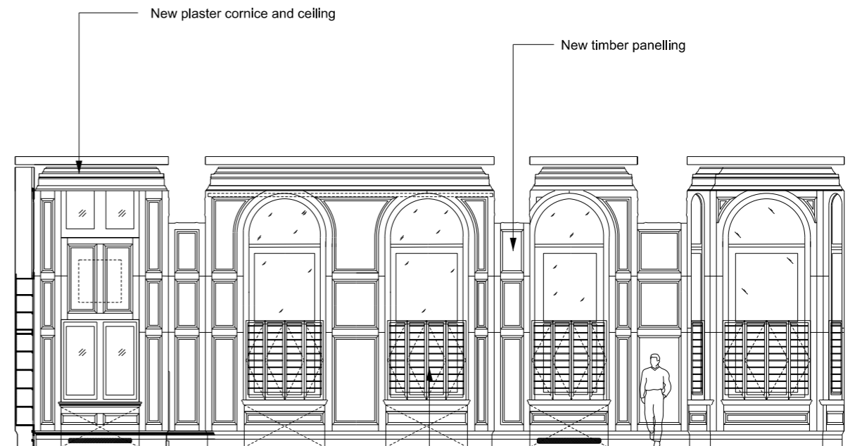
Elevation B
