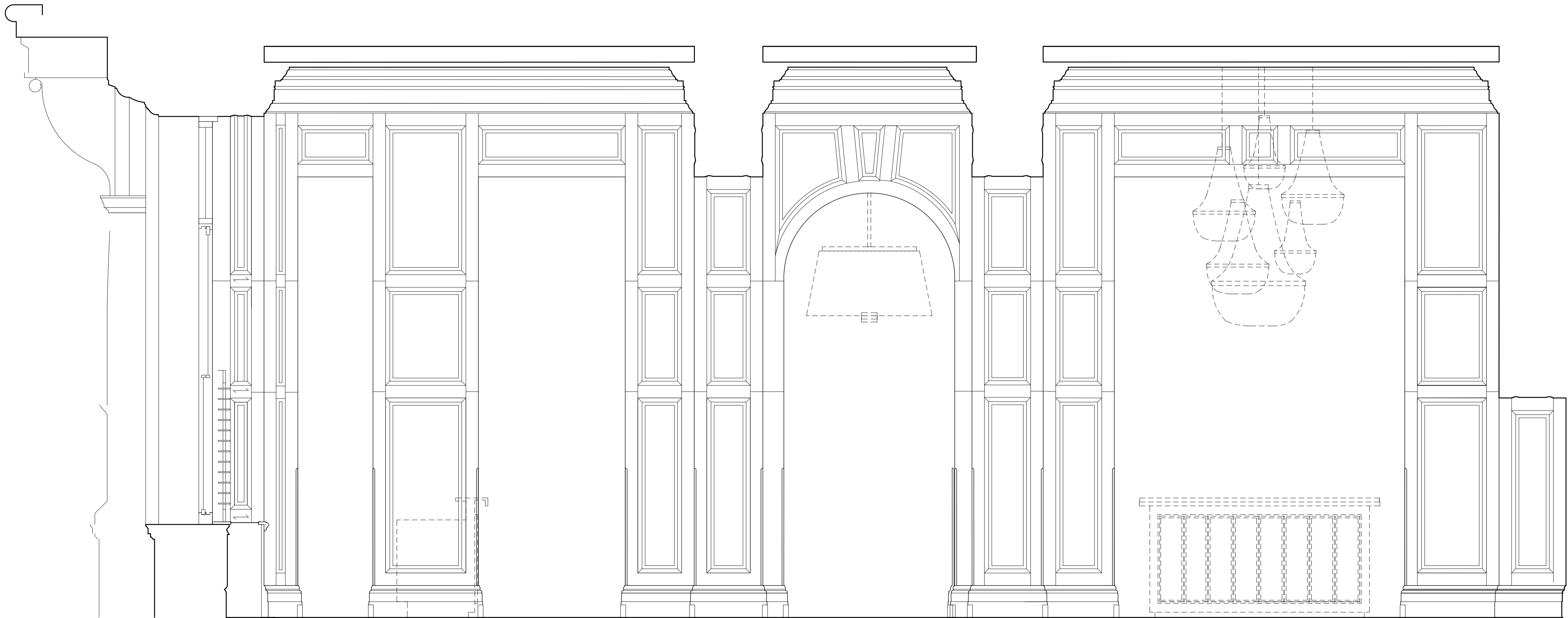
1 ELEVATION D2C scale 1:25
