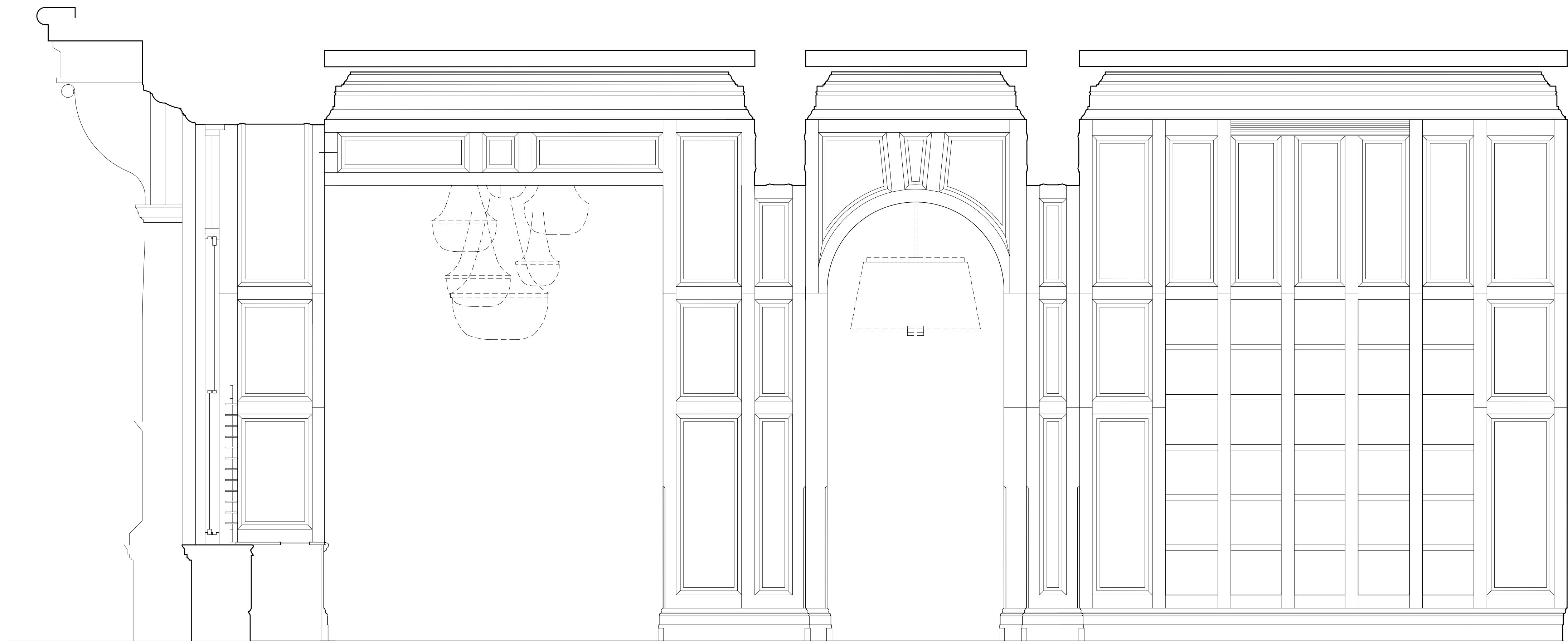
3 ELEVATION D2B scale 1:25
