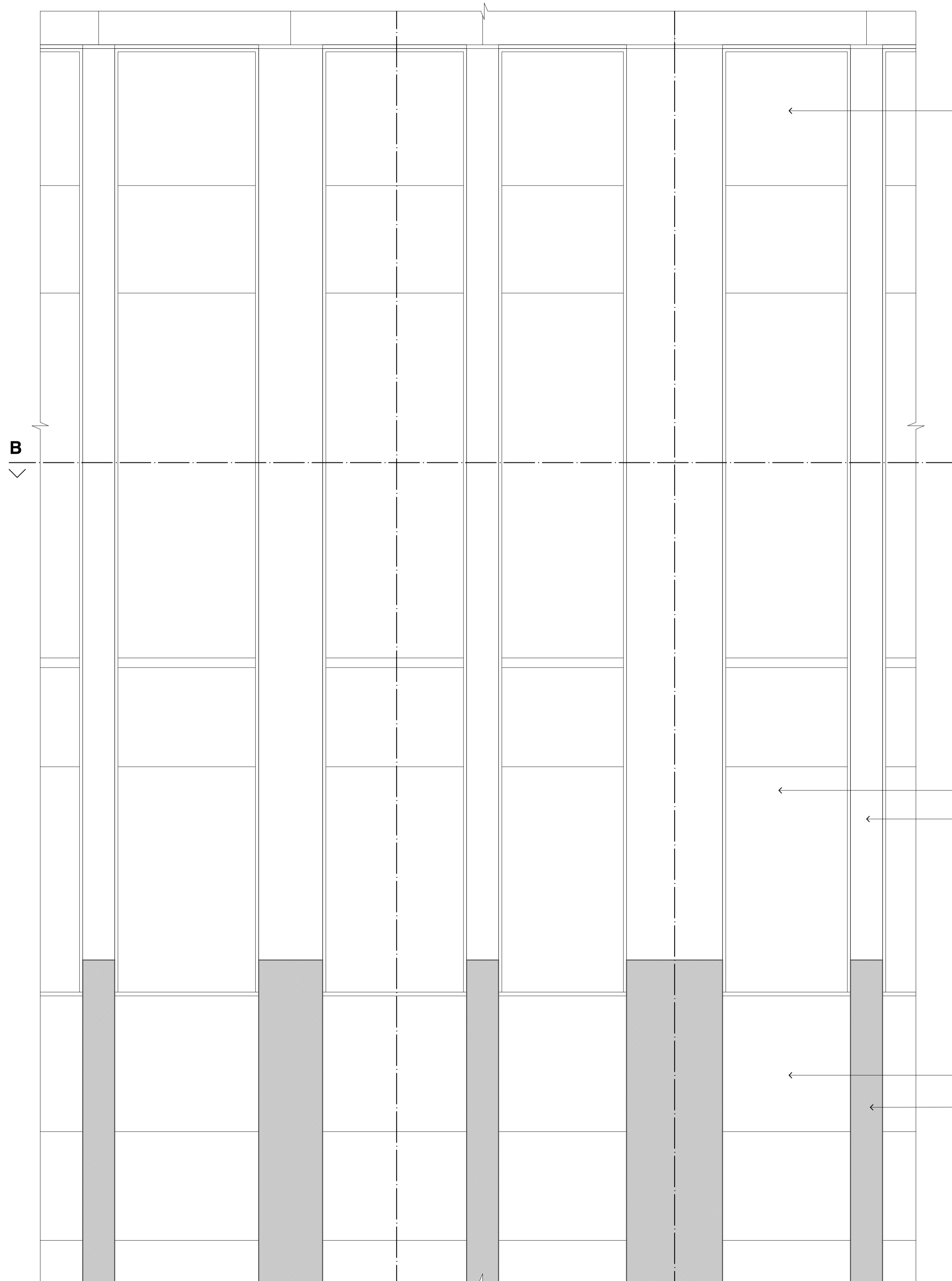
Elevation
