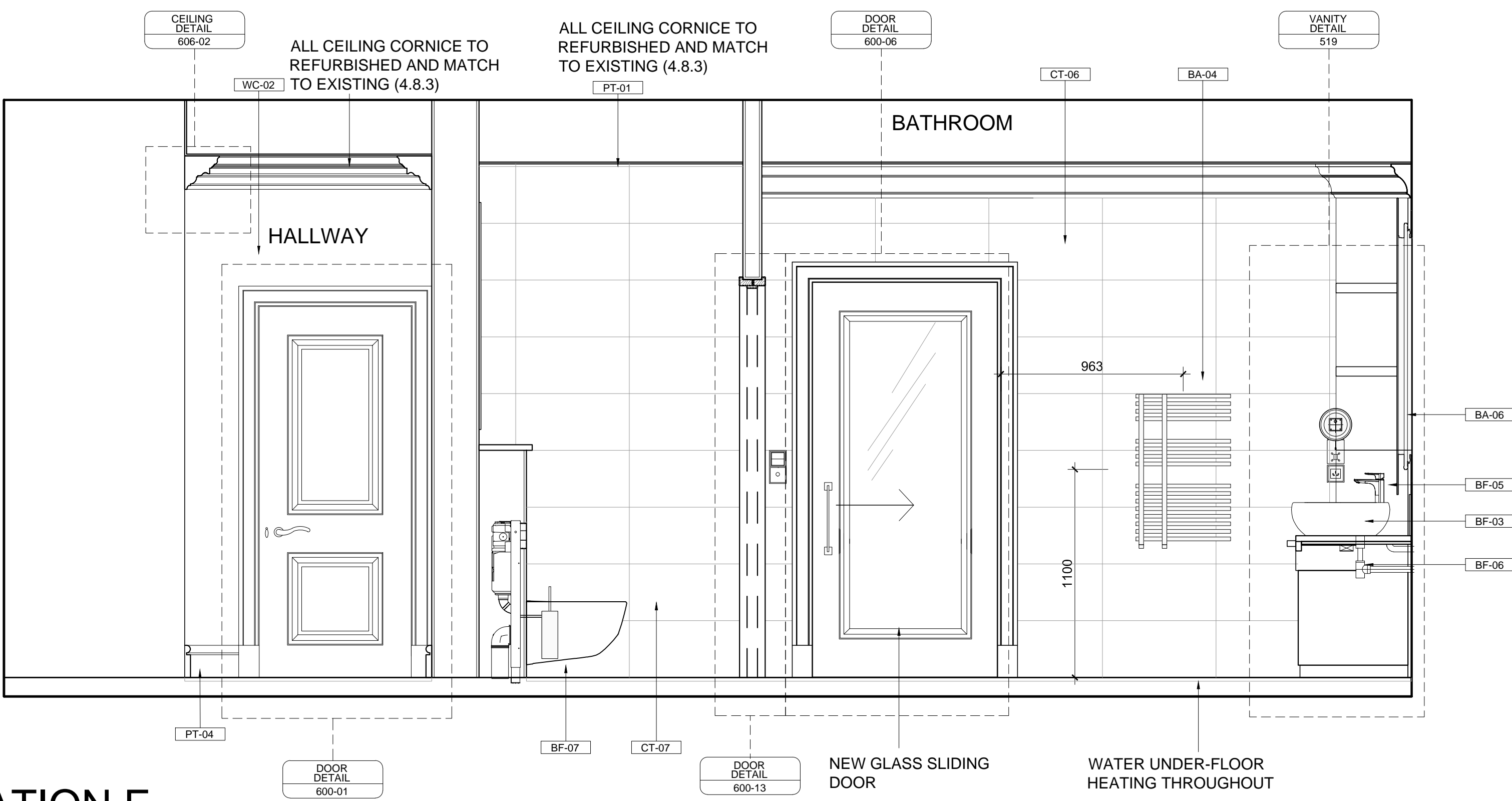
ELEVATION E
