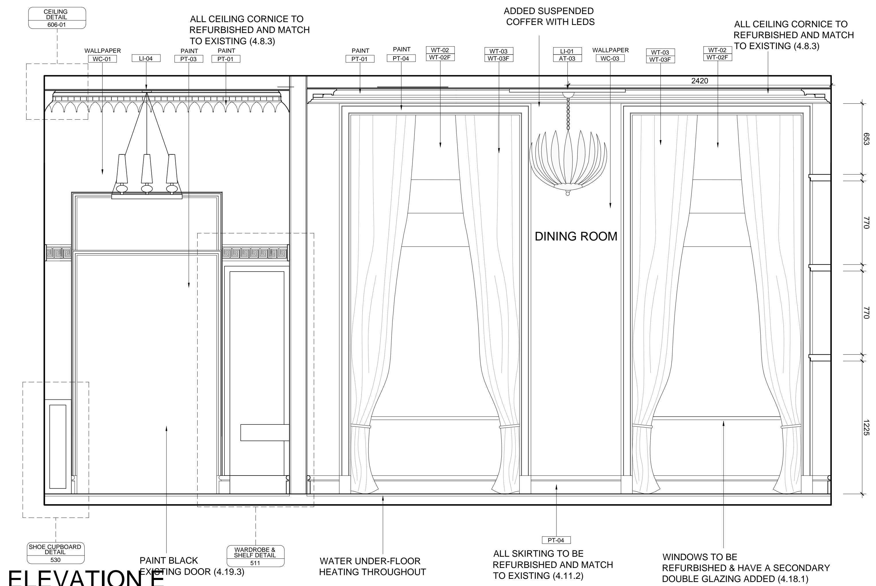
ELEVATION E
