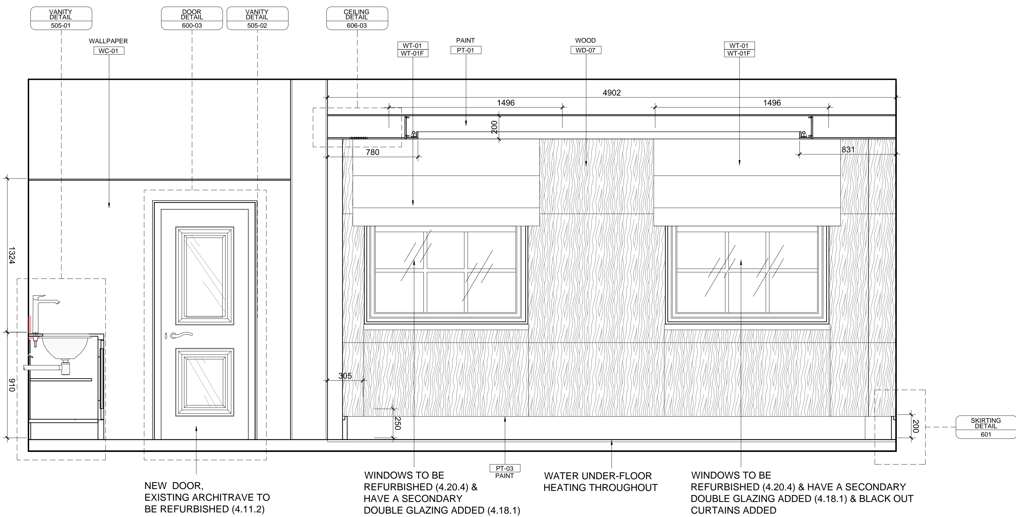
ELEVATION E
