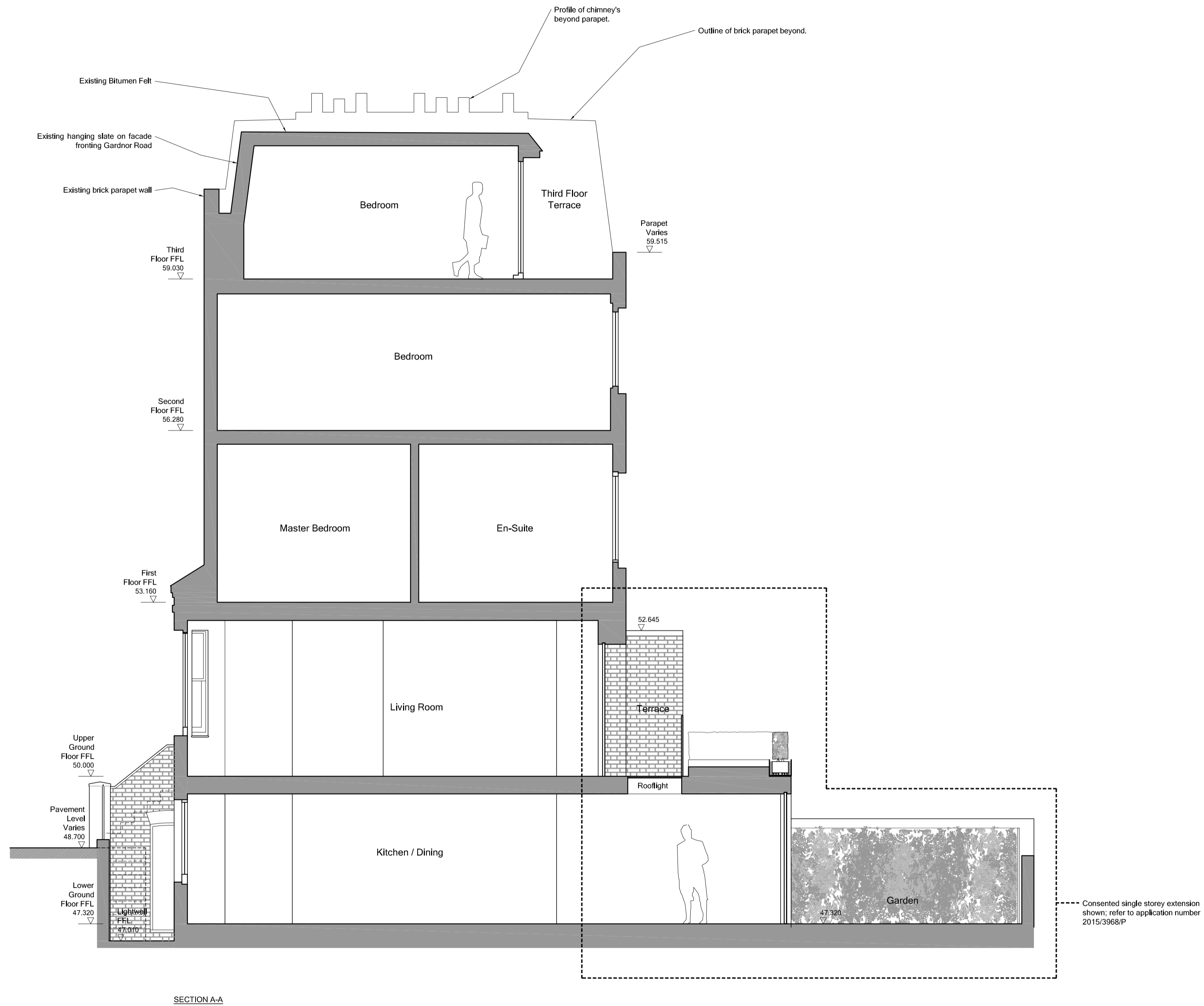
SECTION A-A
