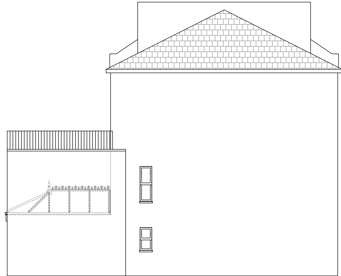
Right Elevation
