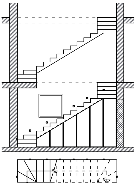
SECTION D-D
