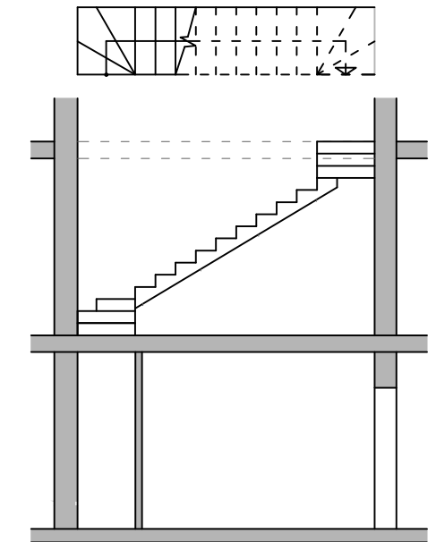
SECTION D-D
