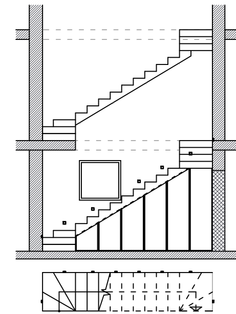
SECTION D-D
