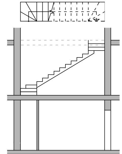
SECTION D-D
