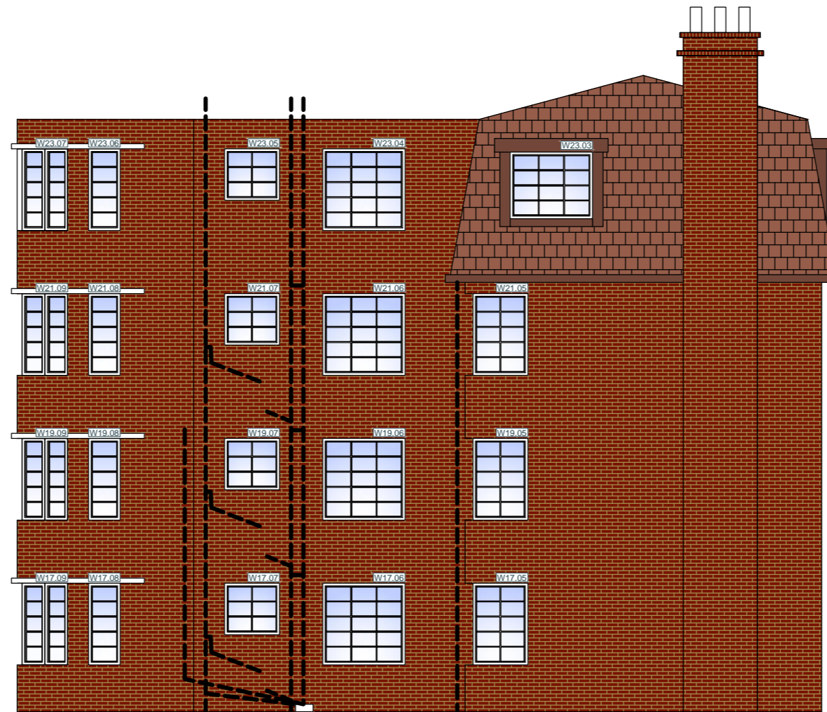
ELEVATION B-B
