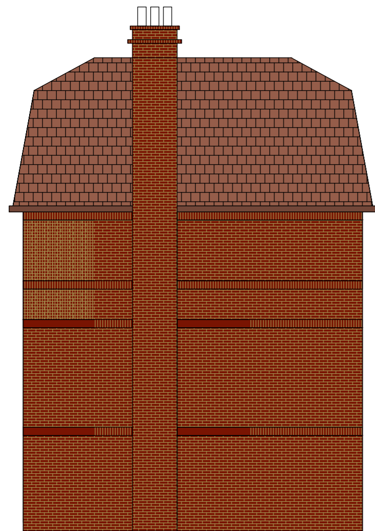
ELEVATION D-D
