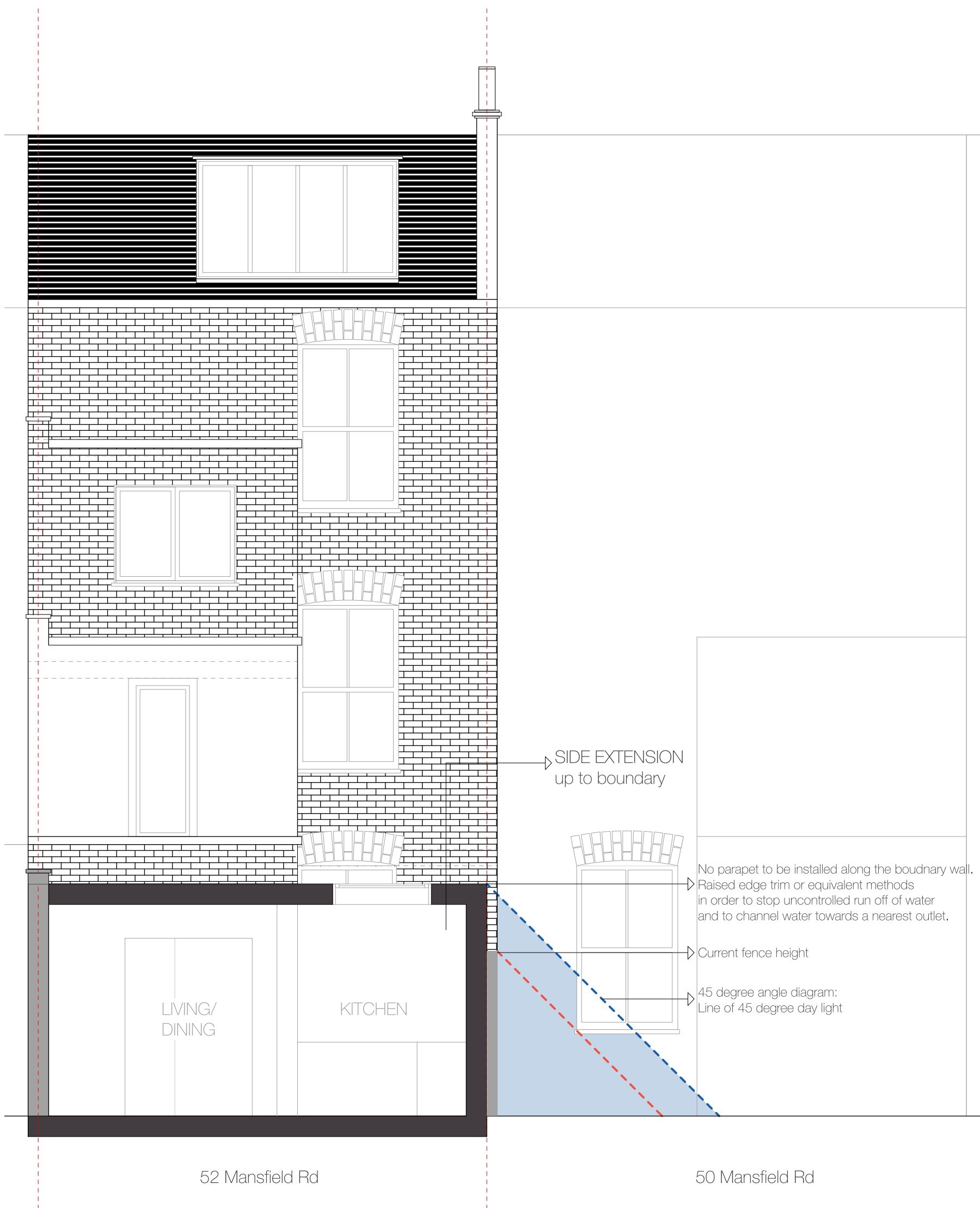
Section a-a
