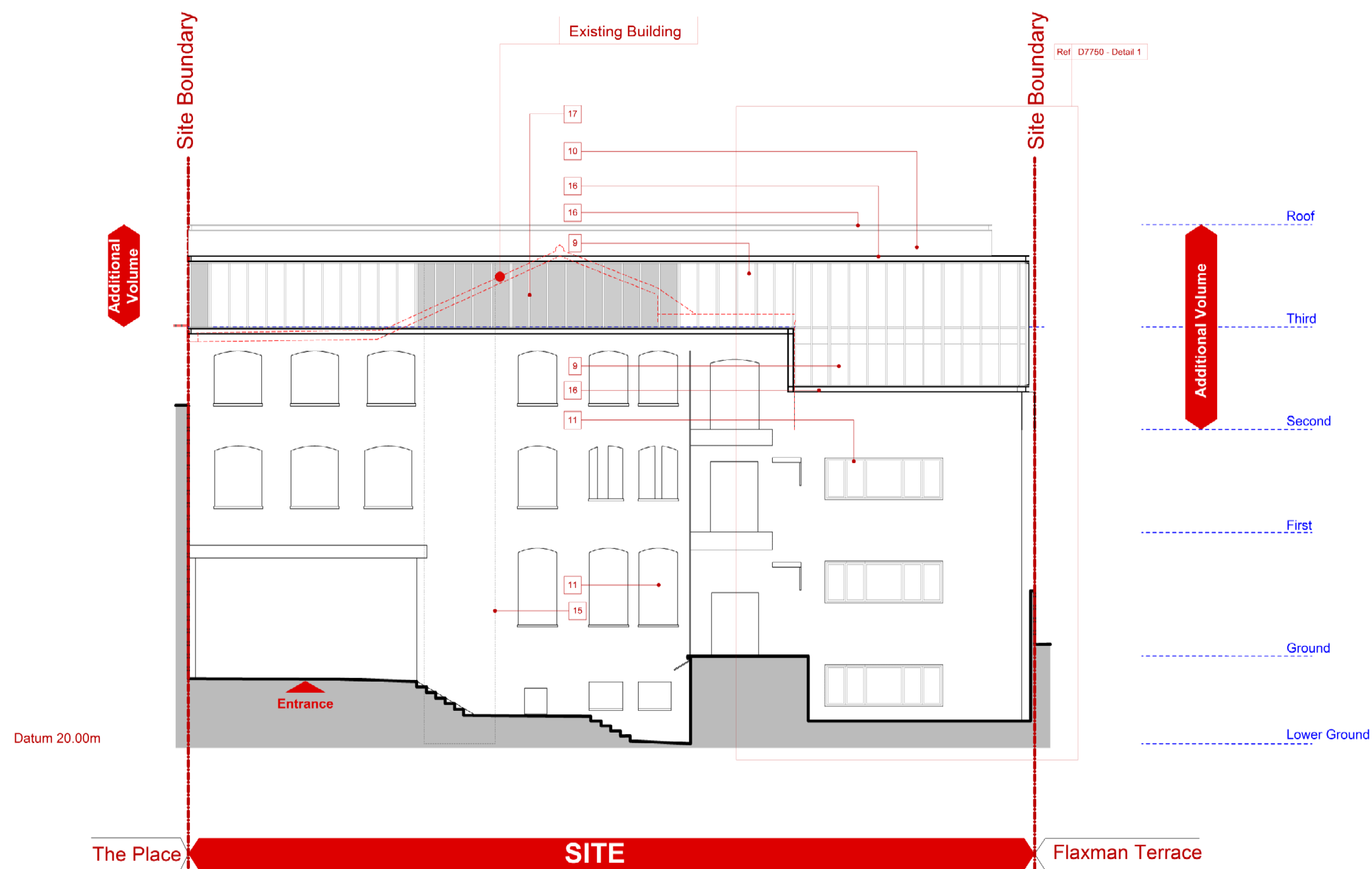
Elevation B-B
