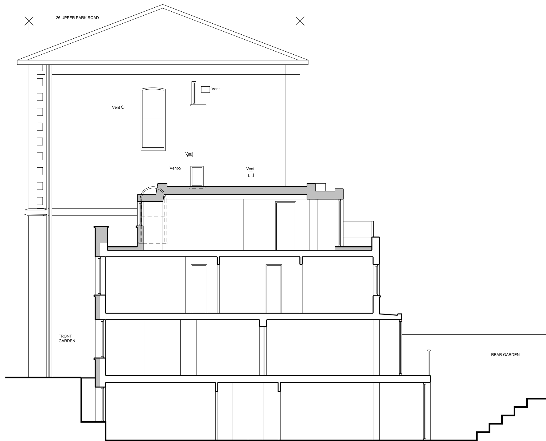
Section A-A
