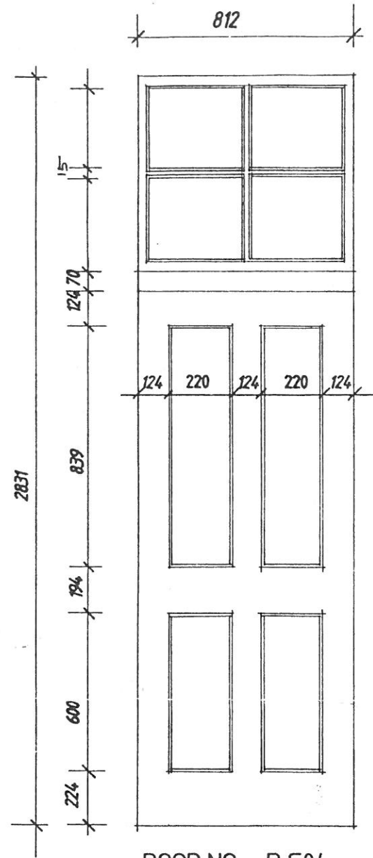
DOOR NO. D G04
