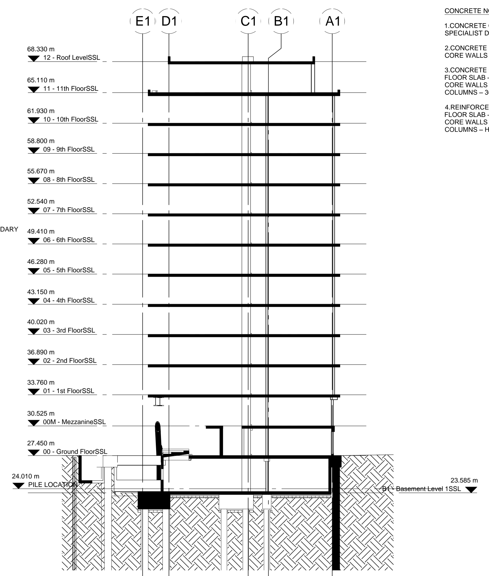
D SECTION D - D 1 : 200
