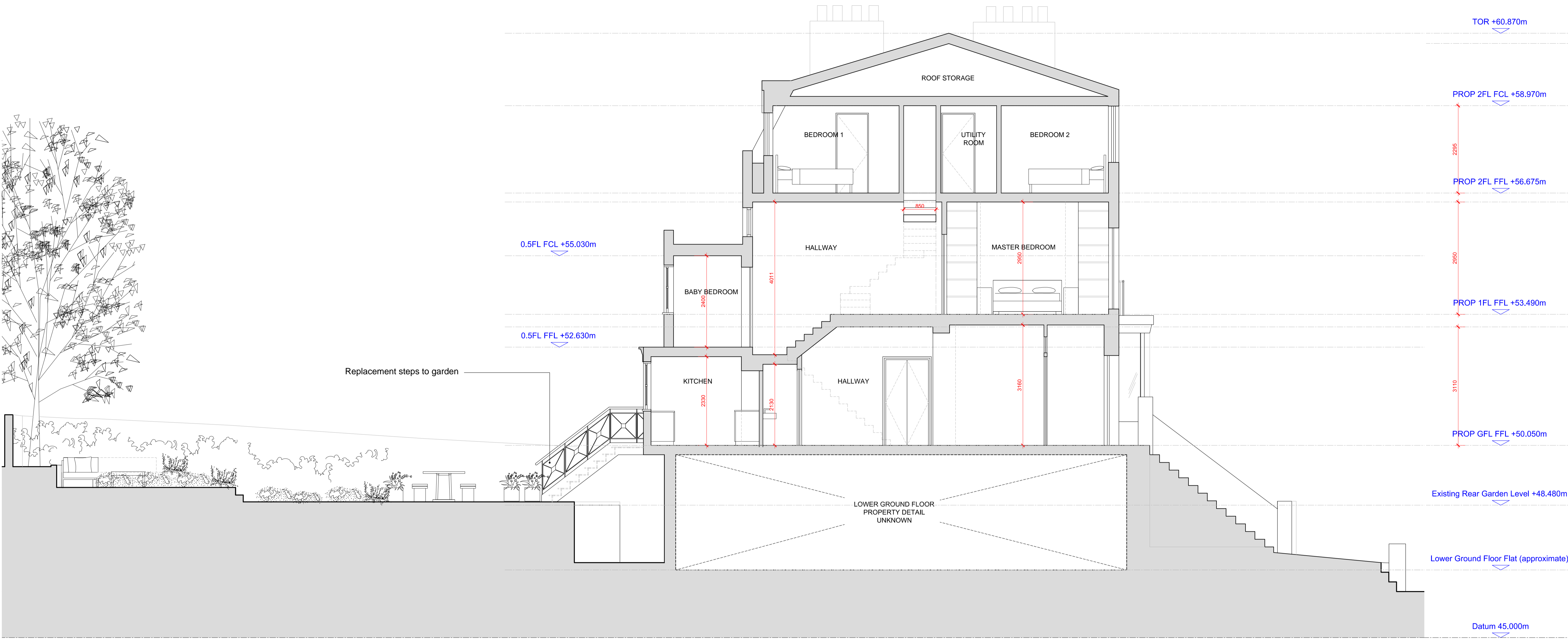
DD SECTION DD 20-212 UPPER PARK ROAD SCALE 1:50
