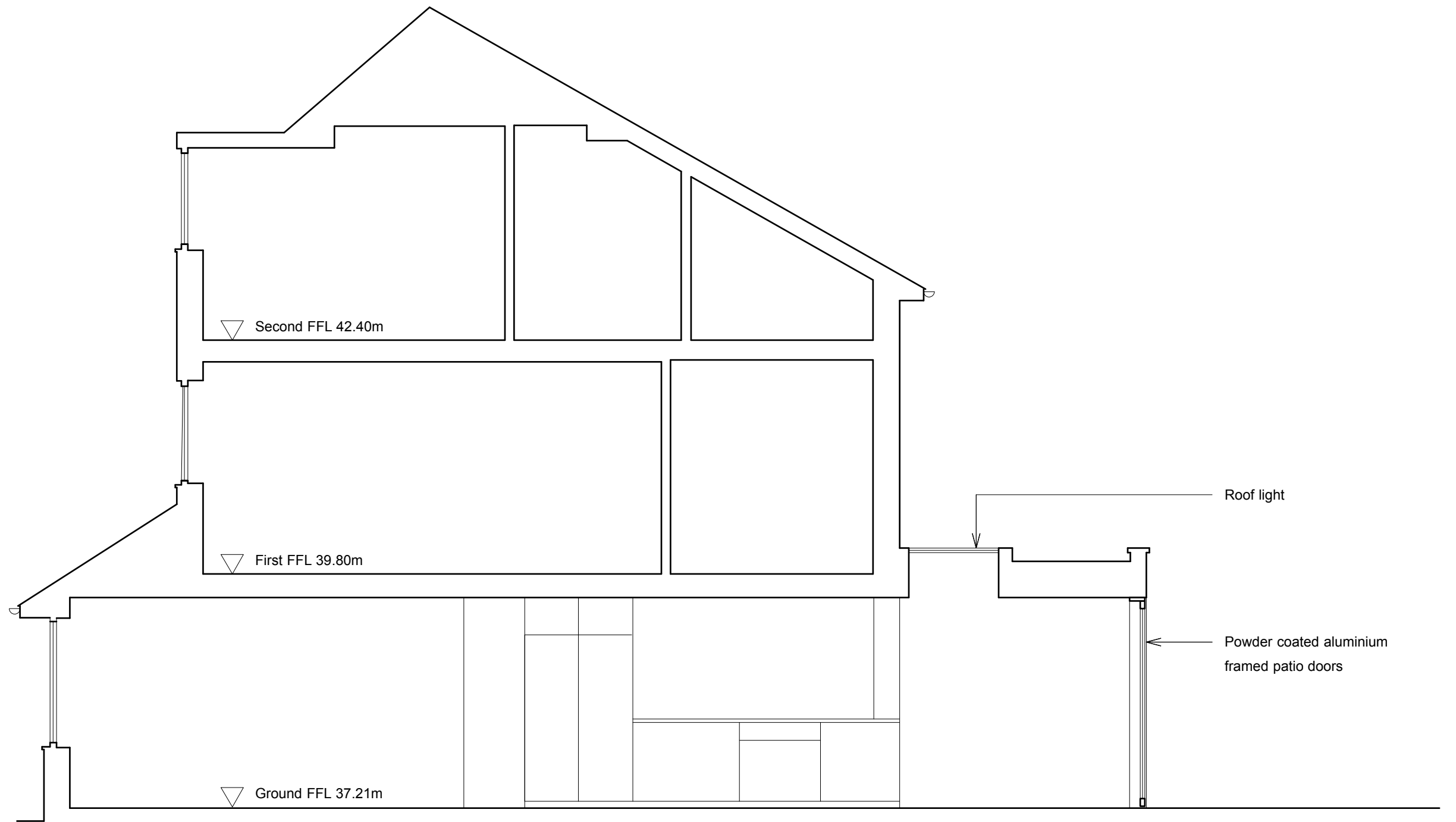
SECTION A-A
