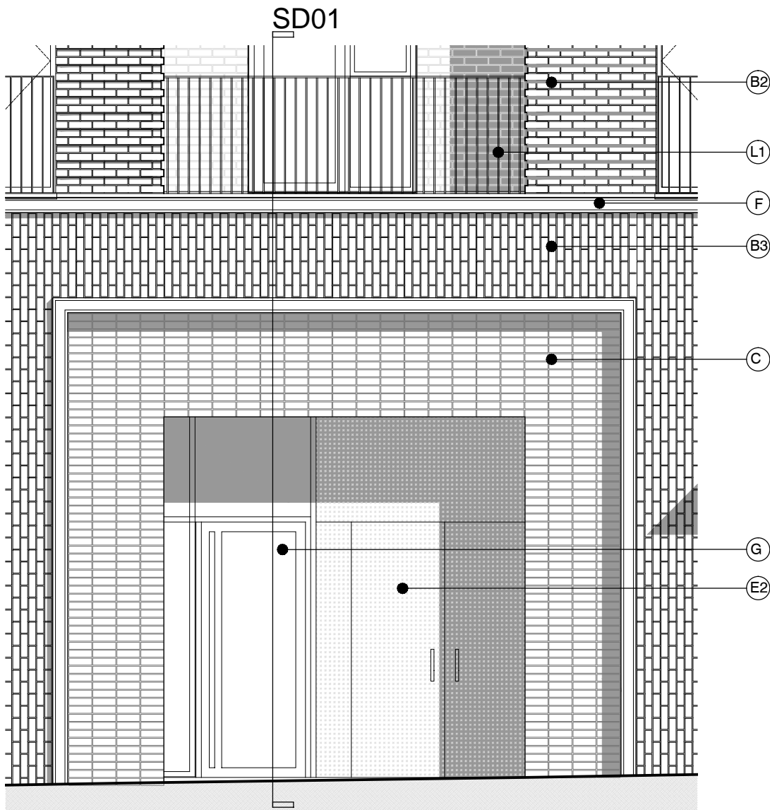
ELEVATION
