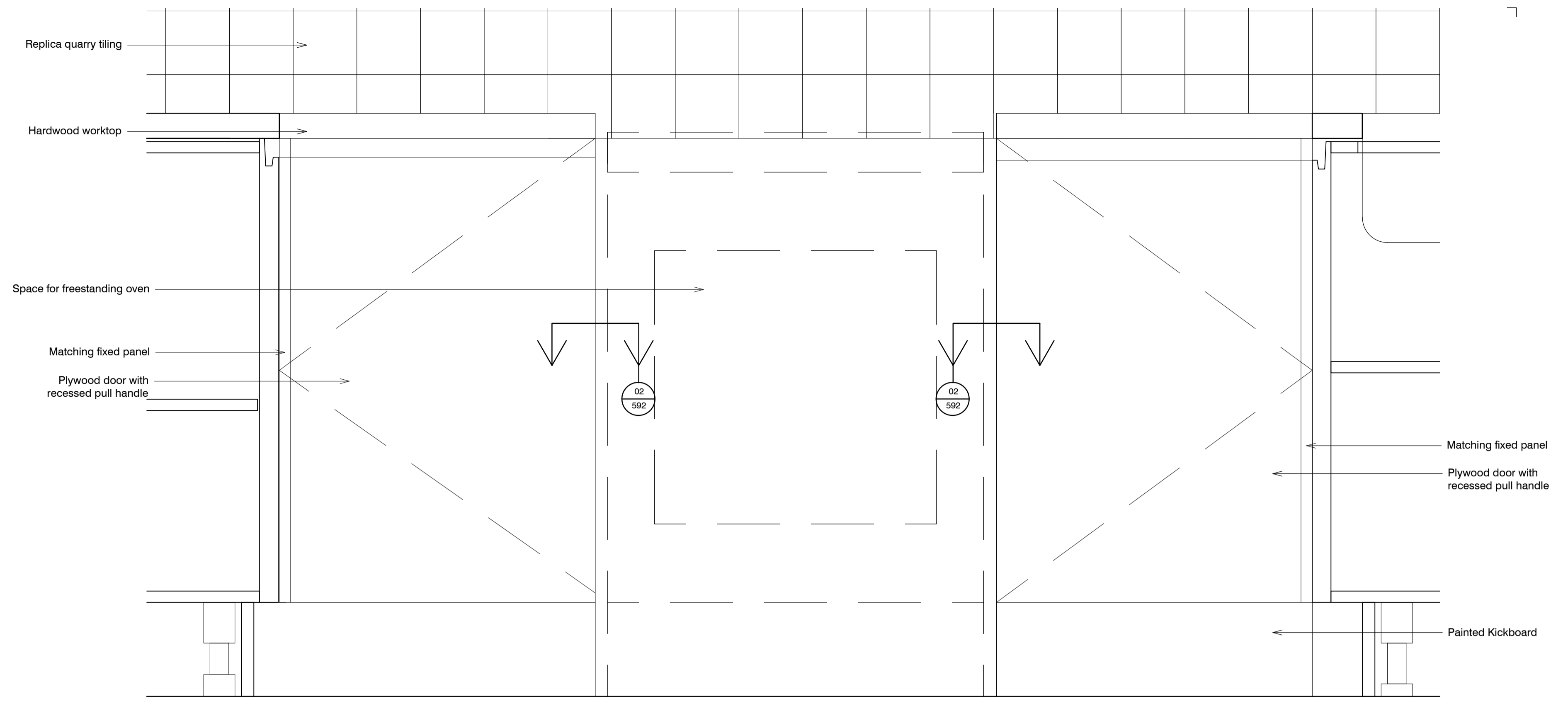
02 Elevation 579
