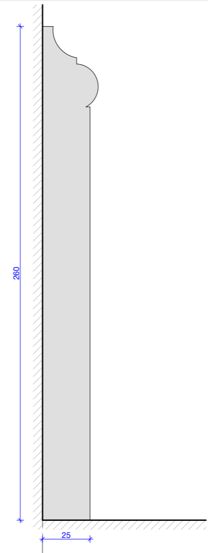
1:2 Door Moulding to match existing
