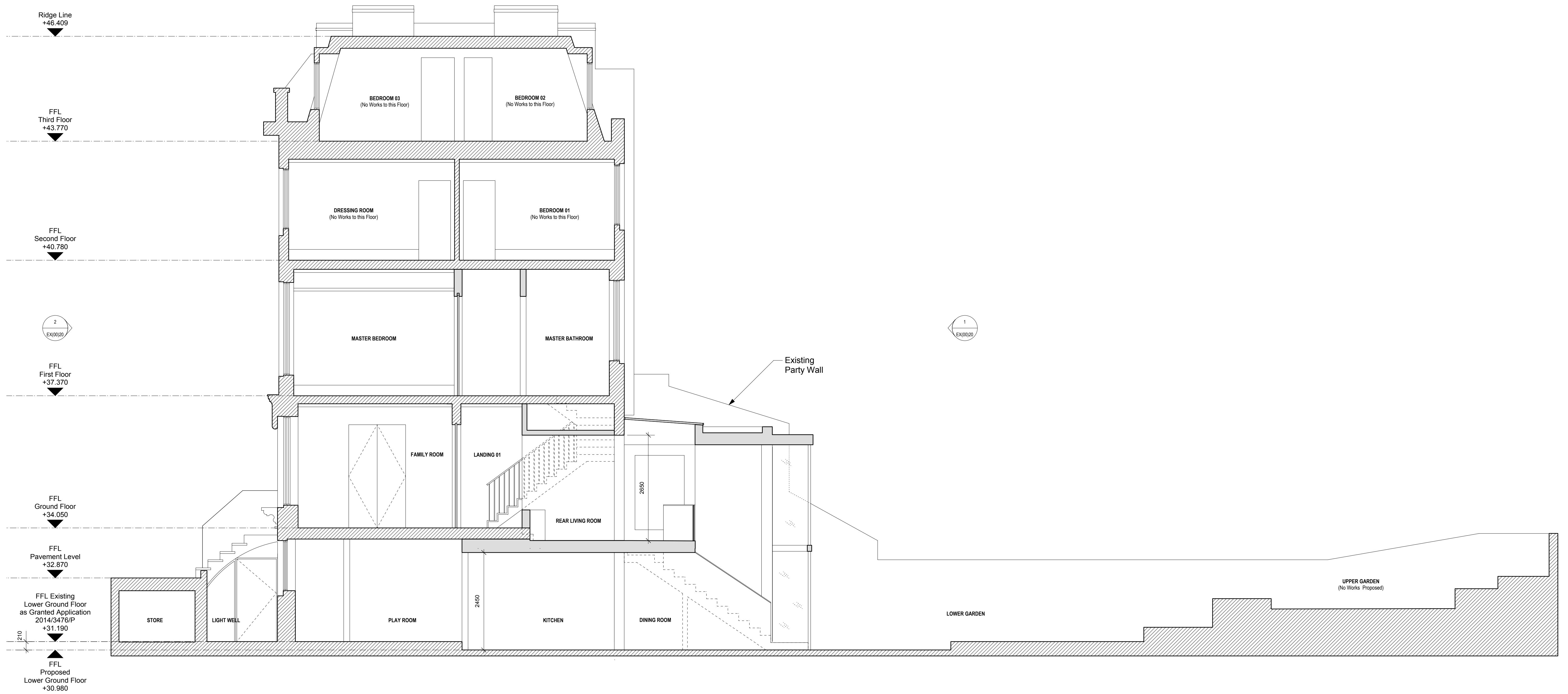
1 Section 01 Scale: 1:50
