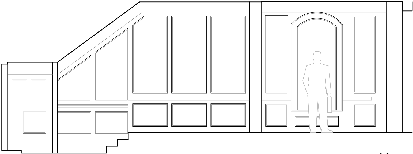
Elevation B 1/50@A3 3 000
