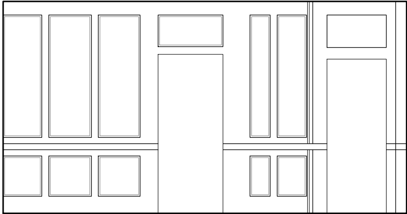
2 000 Elevation C 1/50@A3
