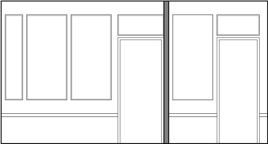
2 Elevation B 000 1/50@A3
