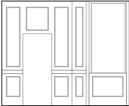
2 000 Elevation C 1/50@A3
