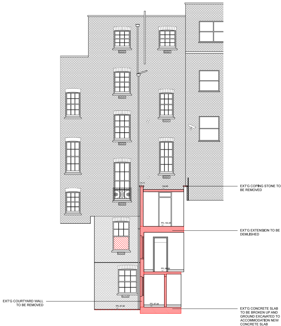
EXISTING SECTION DD
