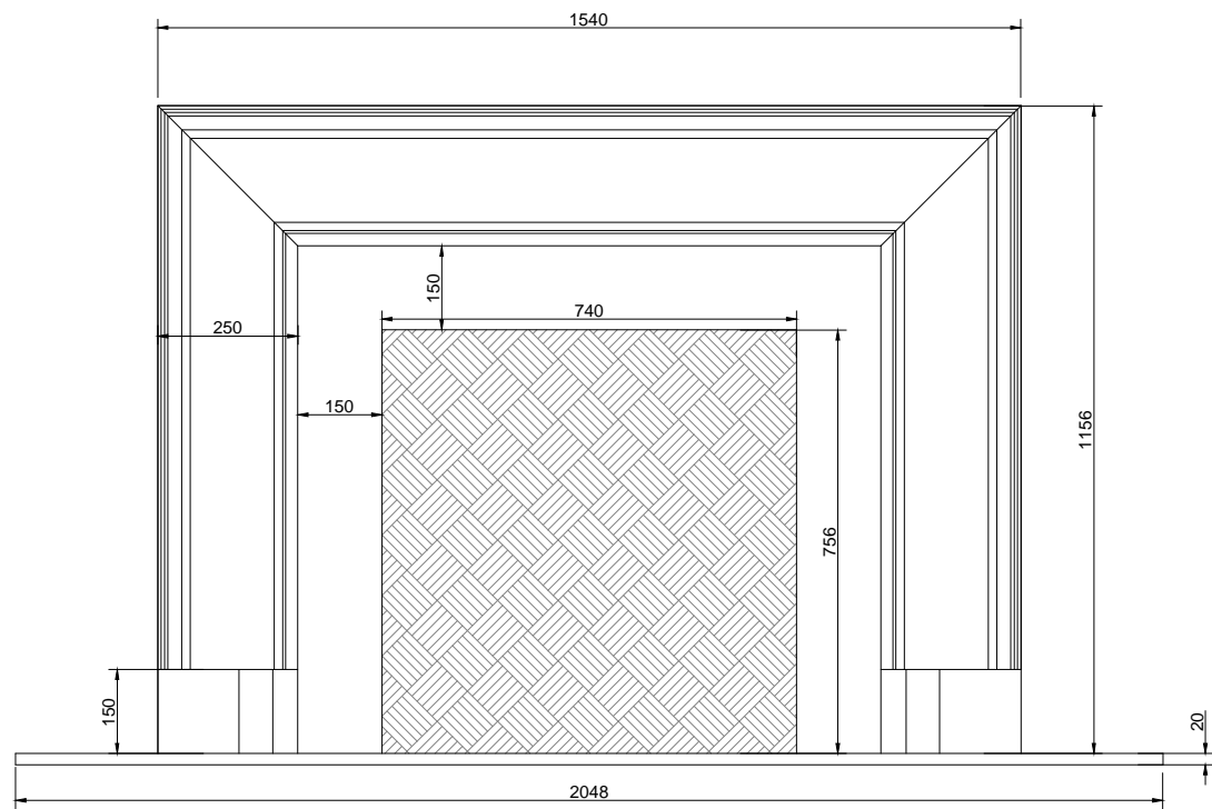
ELEVATION
