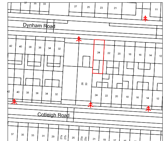
SITE PLAN 1:1250
