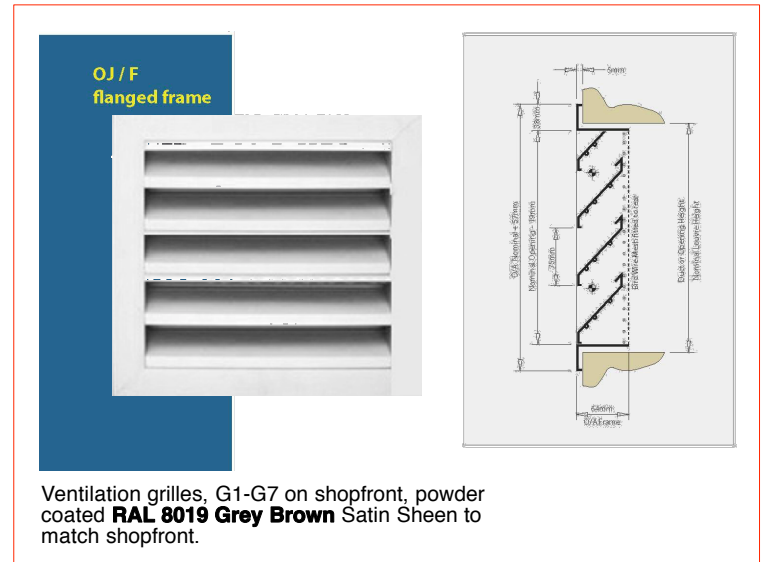
02 OJ/F Flanged Frame Grille n.t.s
