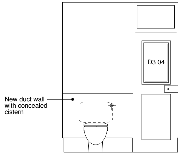
3.05 ELEVATION 1
