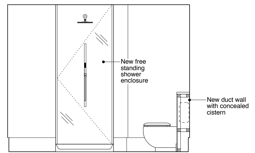
3.05 ELEVATION 4
