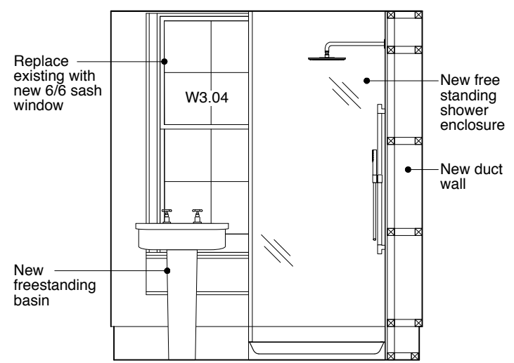
3.05 ELEVATION 3
