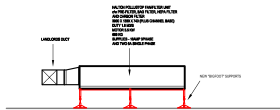
ELEVATION A 1-50
