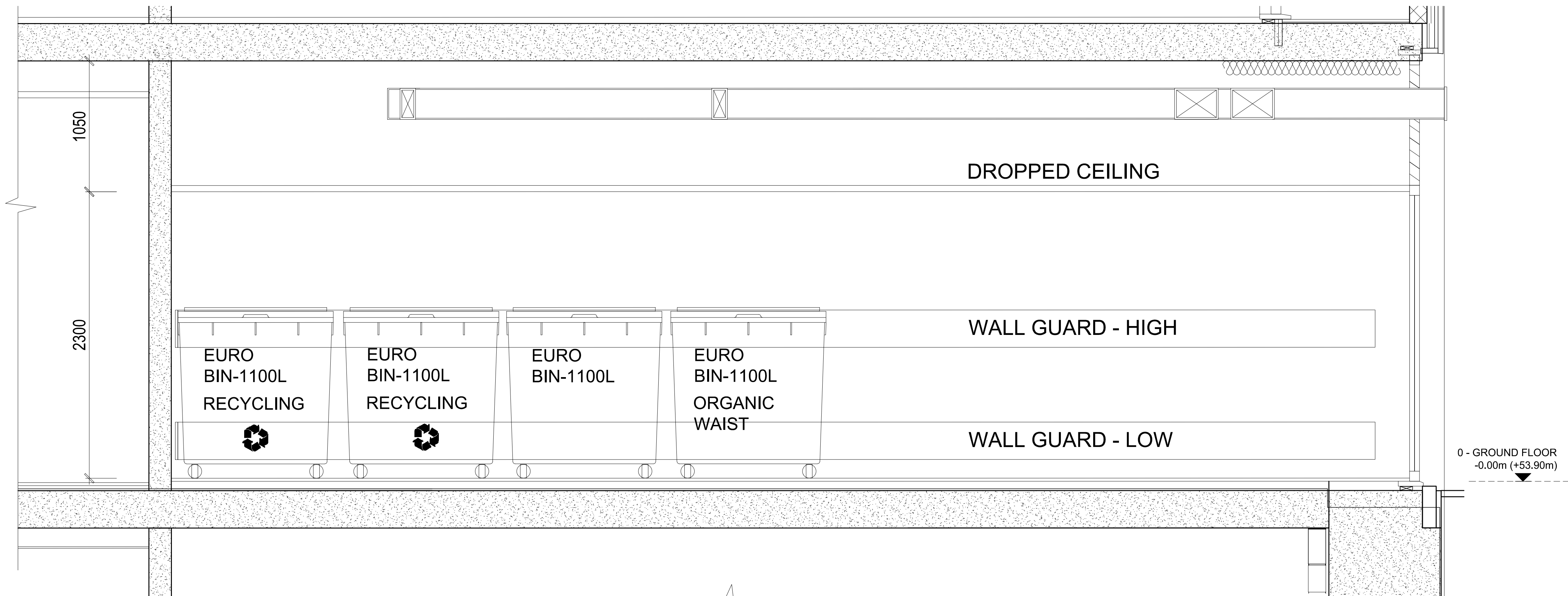
ELEVATION 3
