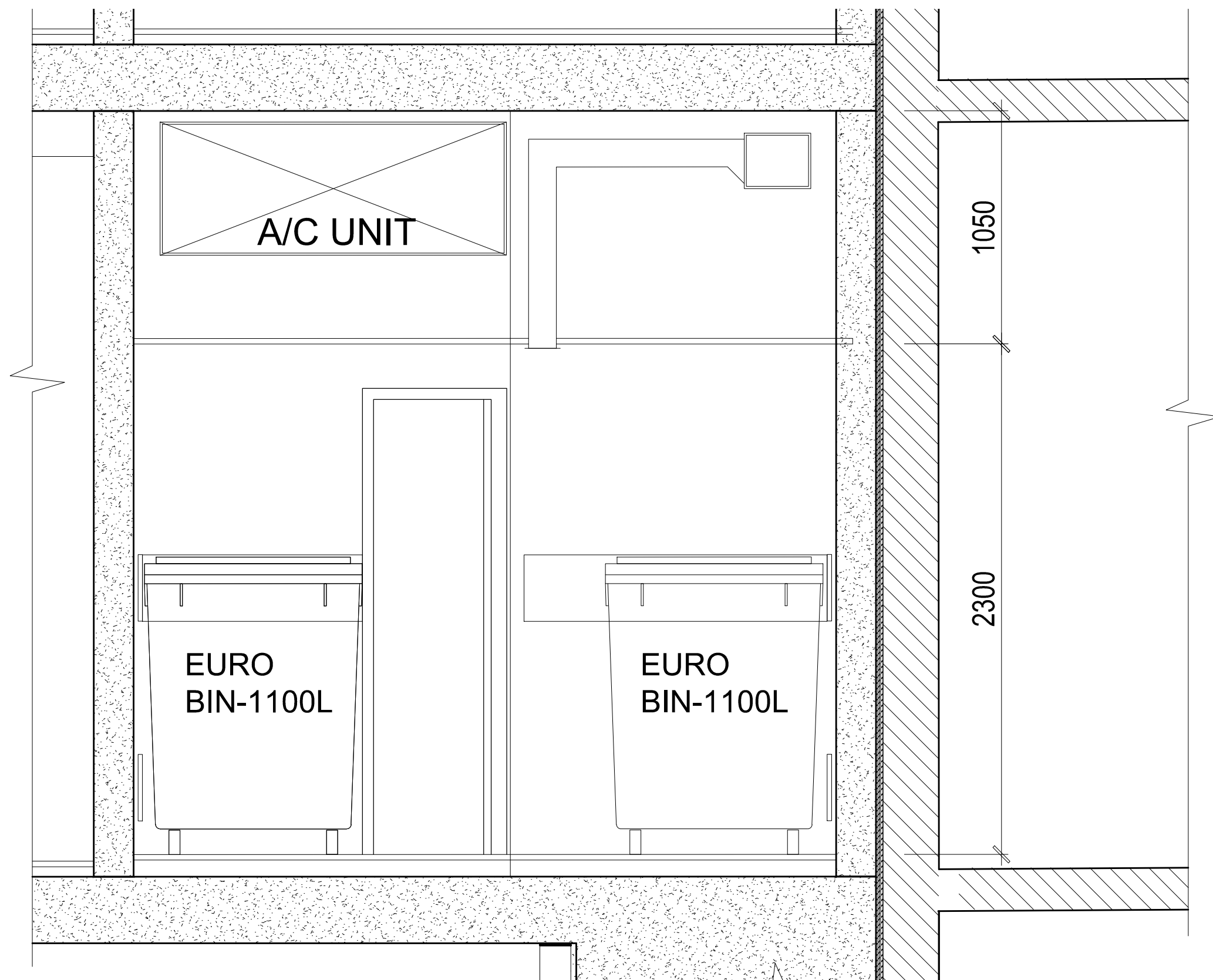
ELEVATION 2
