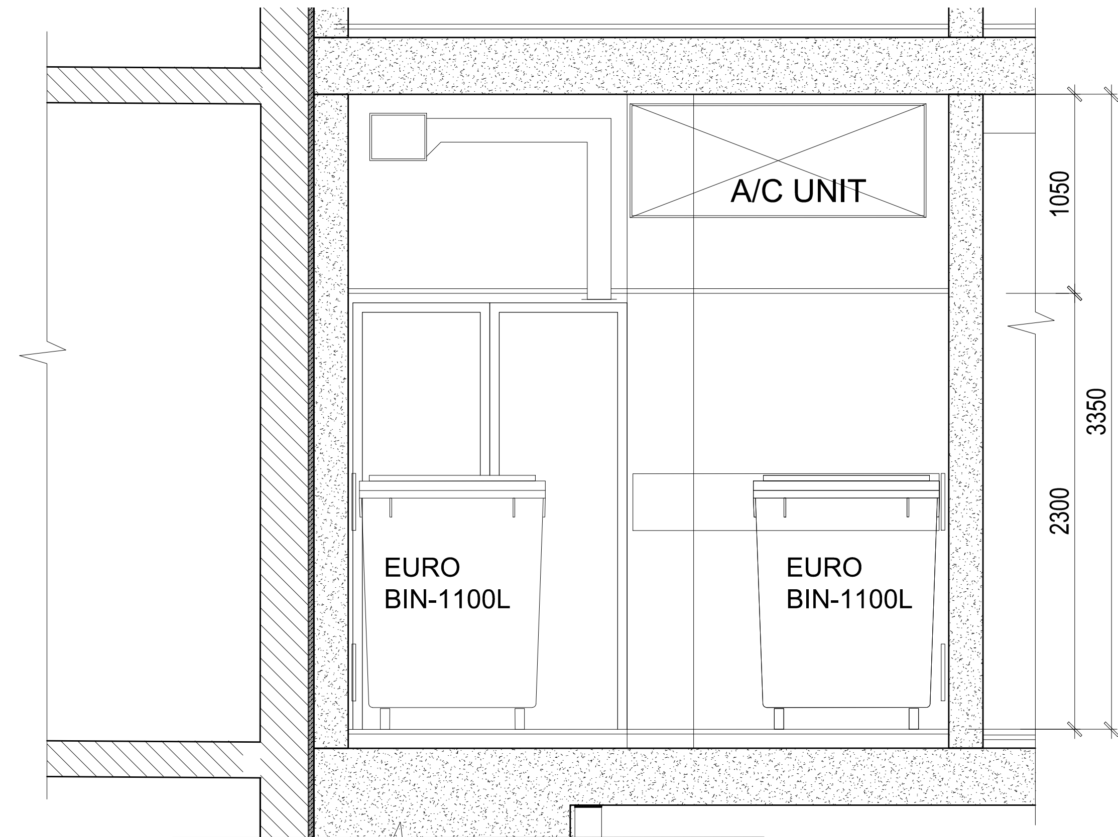
ELEVATION 4
