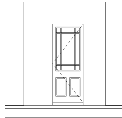
2 Existing Flanking Door Scale @A3 1:50
