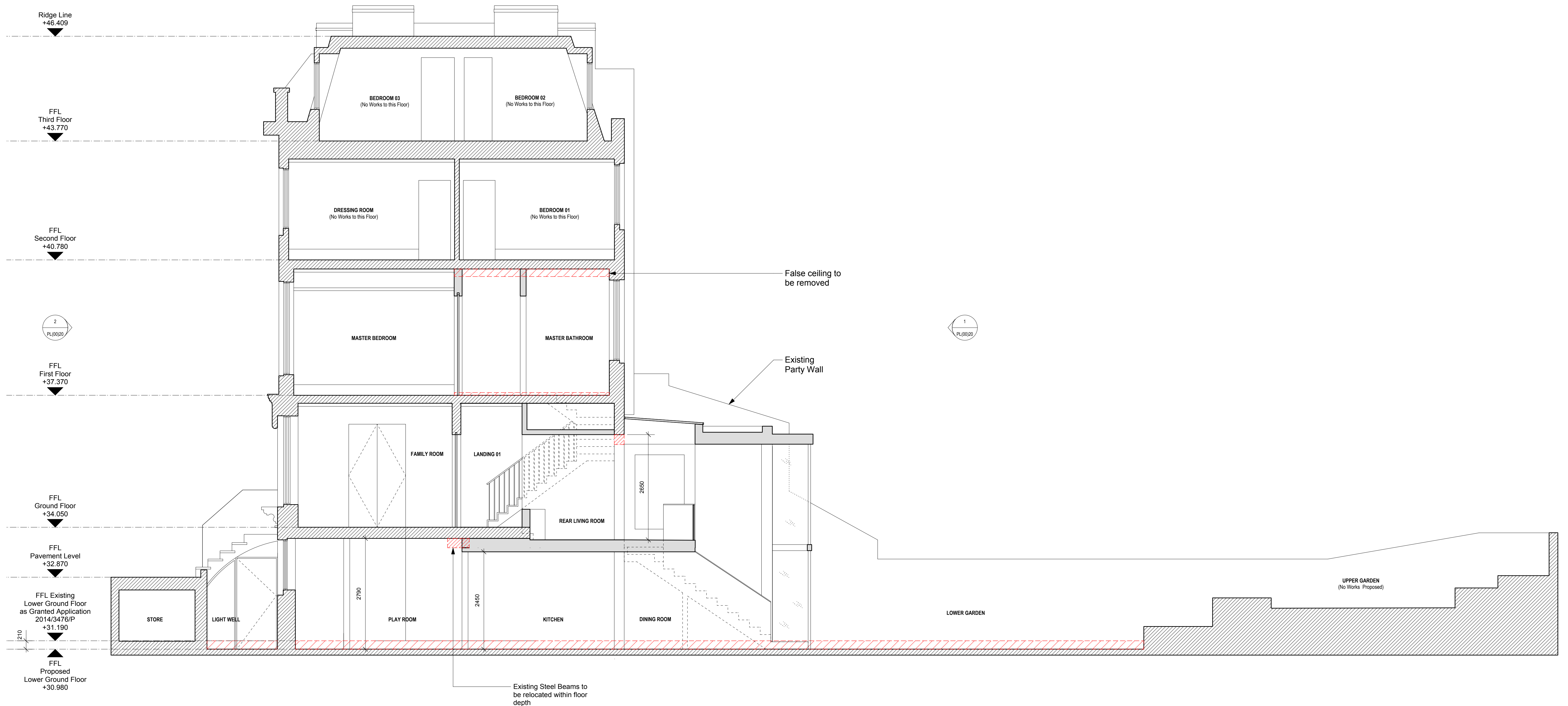
1 Section 01 Scale: 1:50
