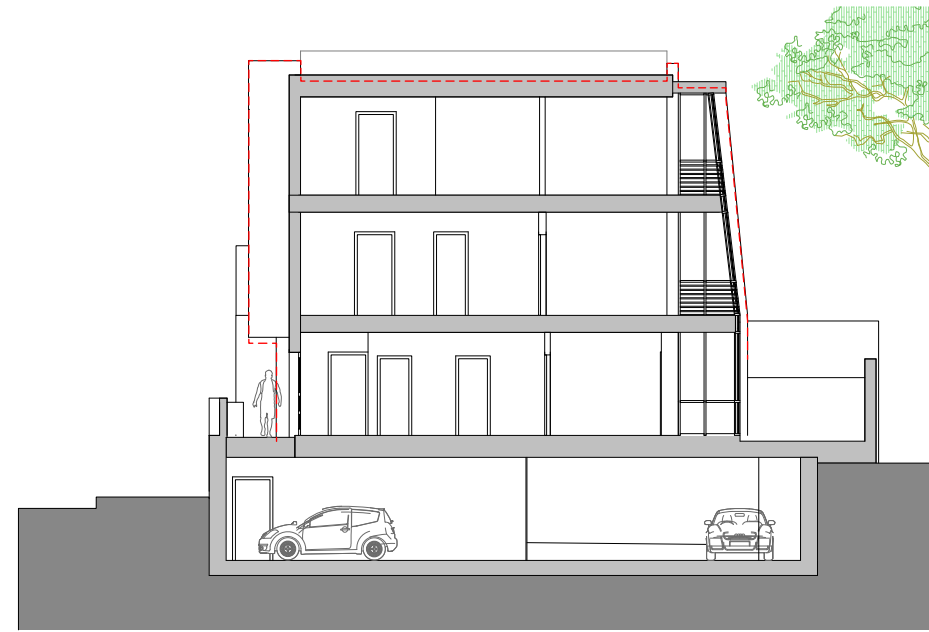
Section BB Scale 1 : 200
