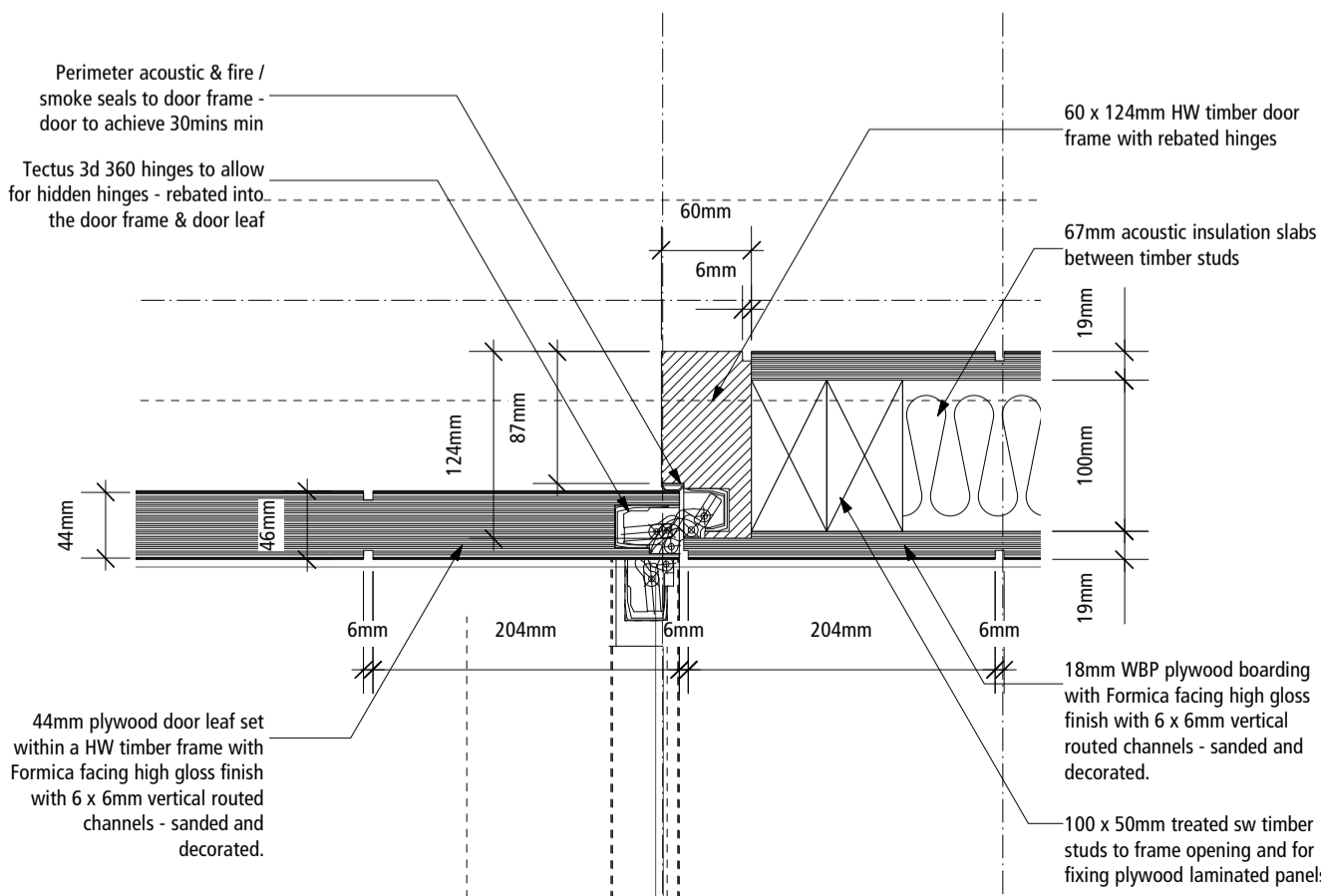
855/01 - JAMB DETAIL @ 1:5
