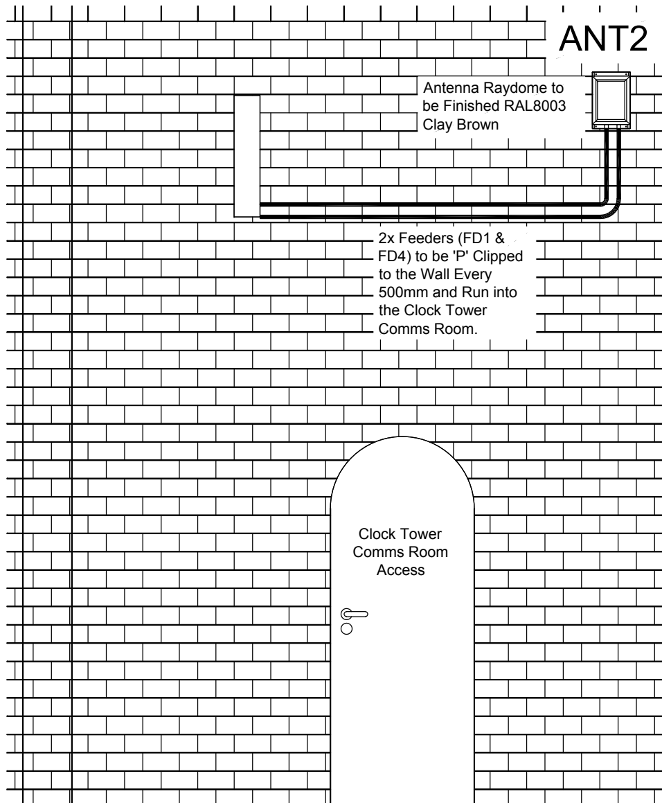
Elevation - 1:20 @ A3
