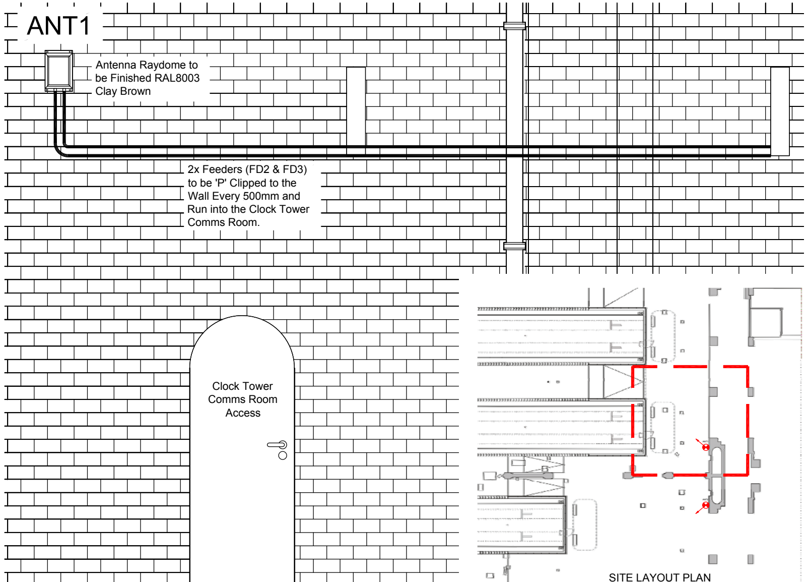
Elevation - 1:20 @ A3
